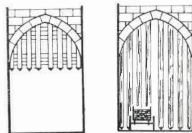
Puertas con rastrillo o con órgano (según Bordejé).
