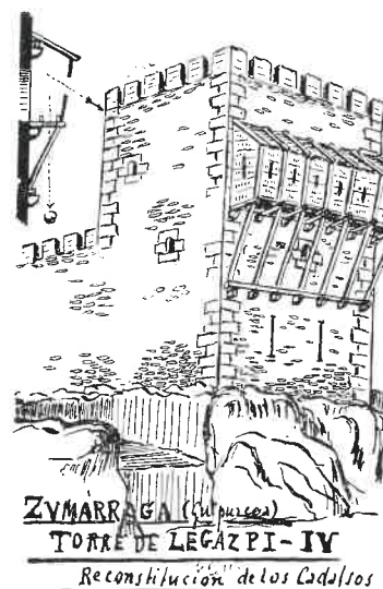
Reconstrucción, hecha por Bordejé, de un cadalso y su empleo.
