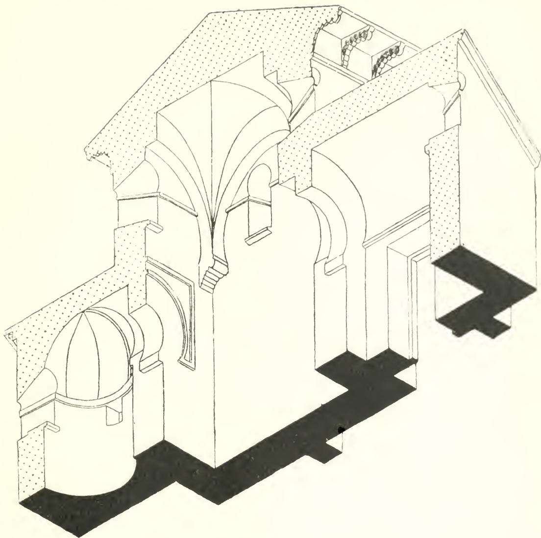
Fig. 122. S. Miguel de Celanova: perspectiva isométrica del edificio
