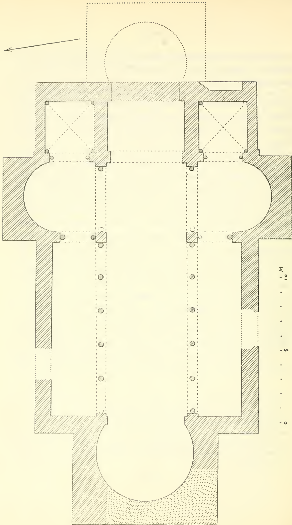
Fig. 75. San Cebrían de Mazote: planta de su iglesia
