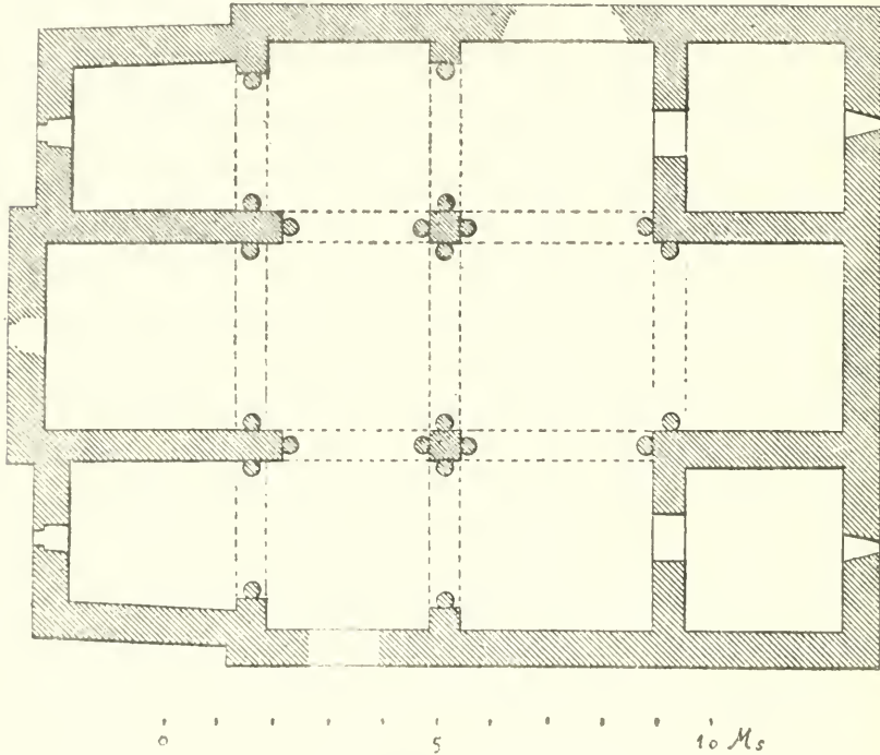
Fig. 134. Sta. María de Lebeña: planta
