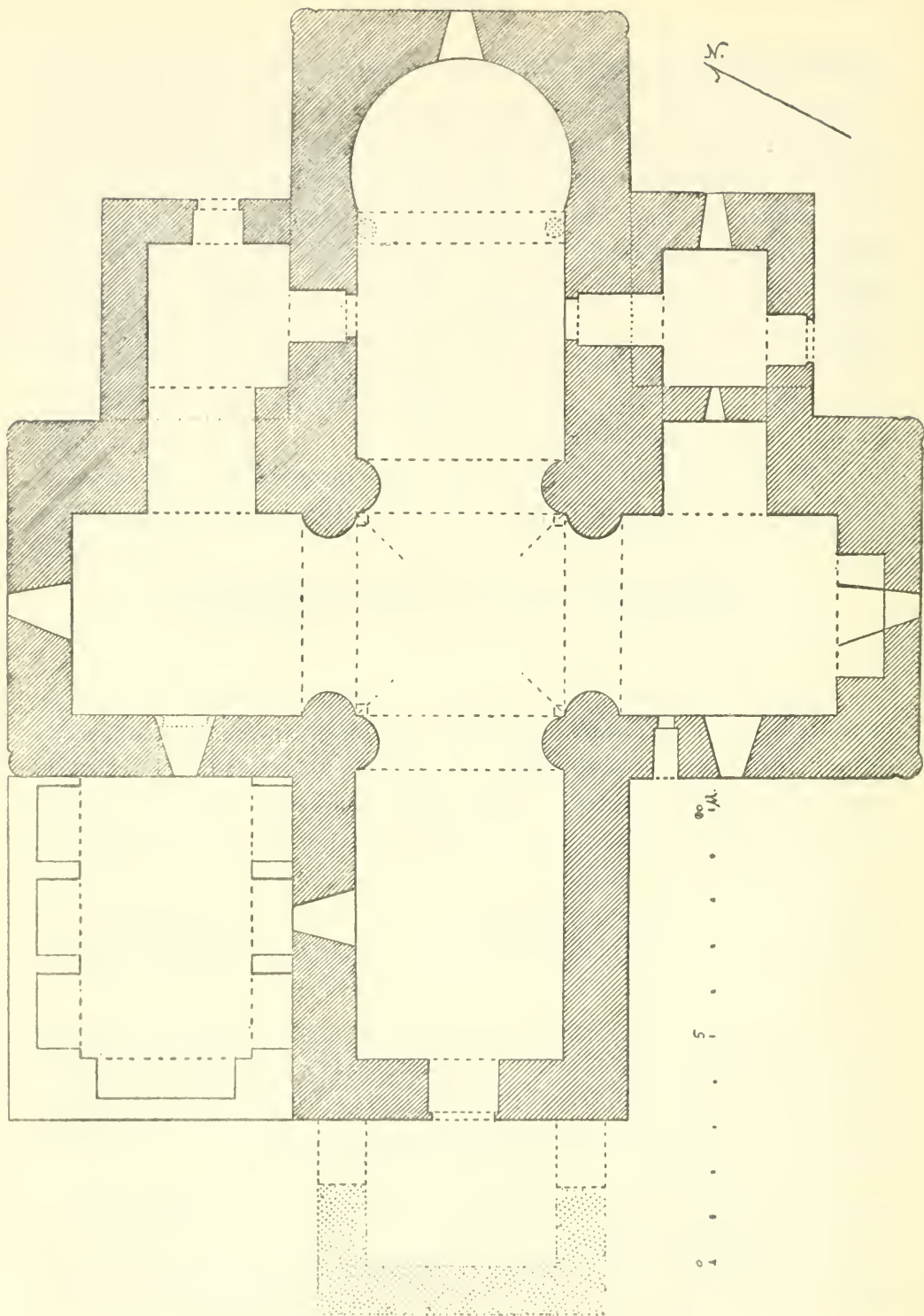
Fig. 4. Planta de Santa María de Melque (Toledo).
