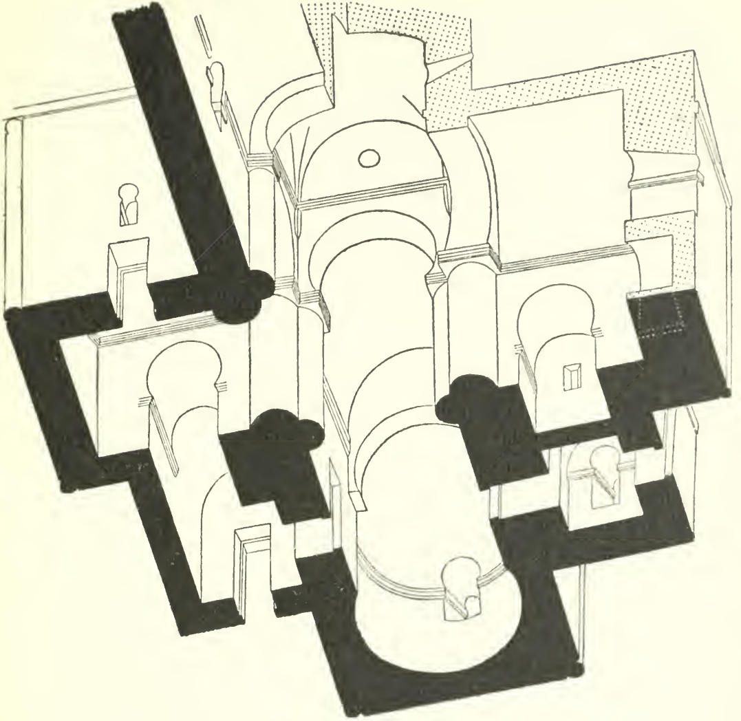
Fig. 7. Perspectiva axonométrica de la iglesia de Melque.
