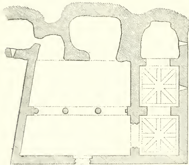
Fig. 107. S. Millán de Suso: planta primitiva restituída
