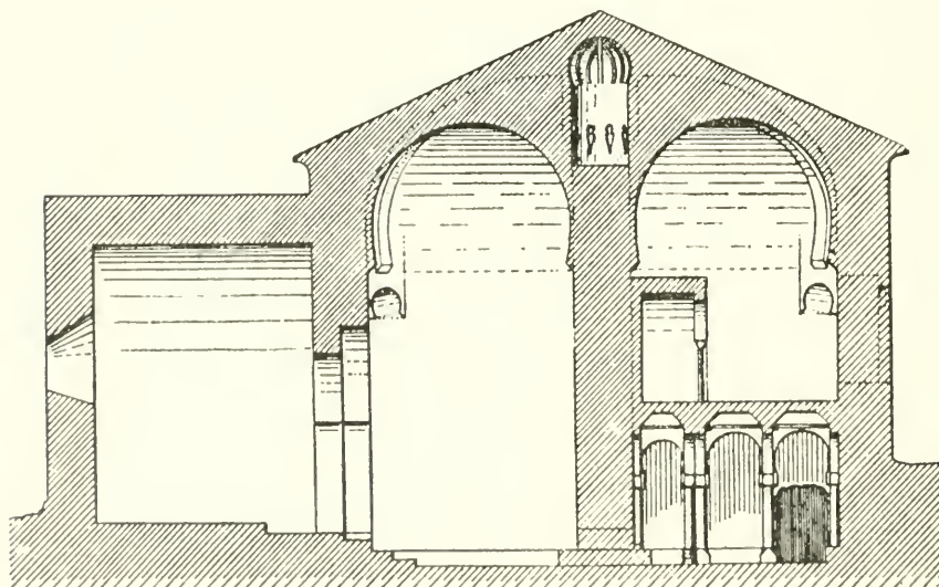
Fig. 182. S. Baudel de Berlanga: sección longitudinal
