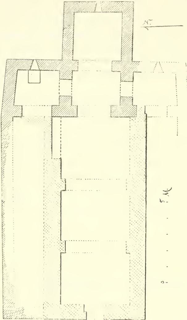
Fig. 25. Santa María de Marquet: planta.
