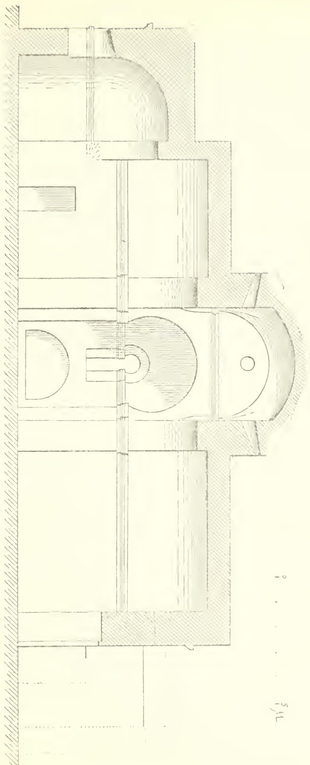
Fig. 5. Sección longitudinal de Santa Maria de Melque.
