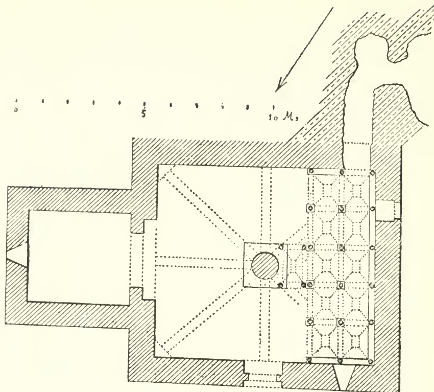
Fig. 181. S. Baudel de Berlanga: planta
