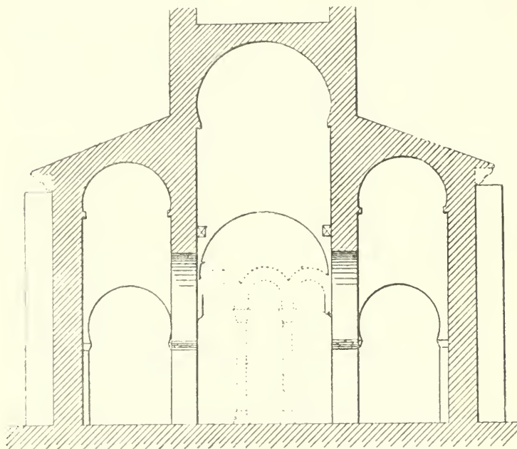
Fig. 93. Bamba: sección transversal, desde la cabecera
